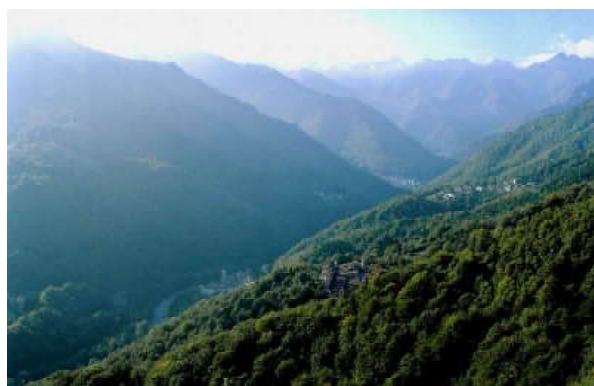
Valle Cervo
